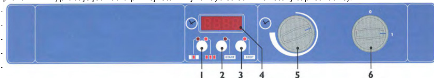
Obr. 1: hlavní vypínač (jednotky s funkcí přizpůsobení teploty), 2 - START, 3 - STOP, 4 - displej, 5 - regulace teploty, 6 - výkon
